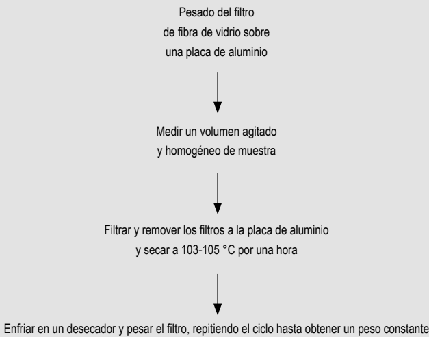
Figura 1 Flujo para la determinación de SST
