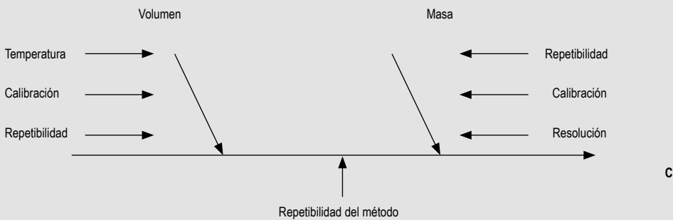
Figura 2 Diagrama causa efecto para la determinación de la incertidumbre
