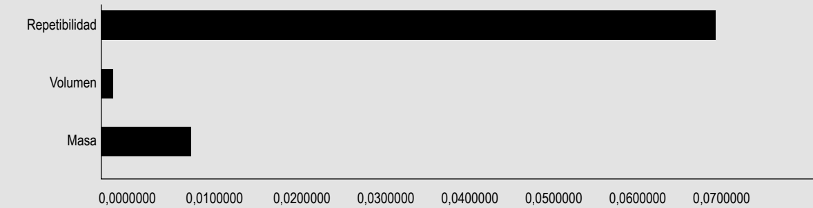
Figura 3 Valores de incertidumbre relativa en la determinación de SST, según el método CITAC/EURACHEM
