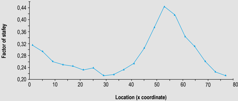
Figura 6 Factor de seguridad crítico para un análisis pseudoestático en el software Slide, versión 5.014
