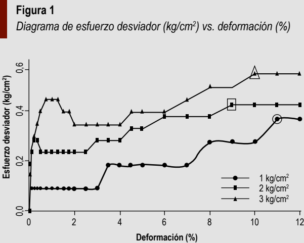
Nota. La figura muestra el diagrama de dispersión de los esfuerzos desviadores y deformaciones a presiones de celda de 1, 2 y 4 kg/cm² (CISMID-UNI, 2019).
