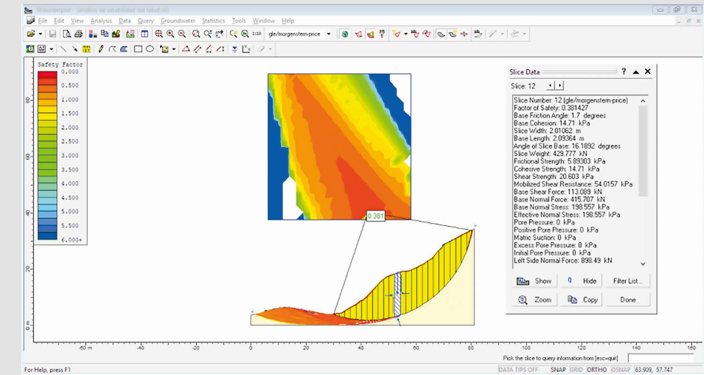
Nota. La figura muestra el cálculo del factor de seguridad obtenido por la técnica de dovelas para un análisis estático.
