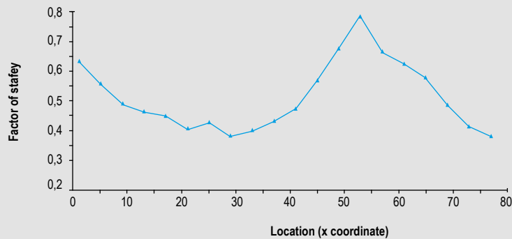
Figura 5 Factor de seguridad crítico para un análisis estático en el software Slide, versión 5.014
