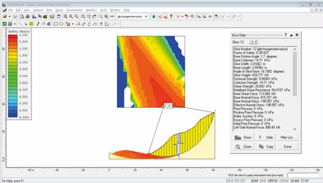
Figura 4 Cálculo del factor de seguridad para un análisis pseudoestático en el software slide, versión 5.014
