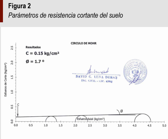
Nota. La figura muestra los parámetros de resistencia cortante del suelo. (CISMID-UNI, 2019).
